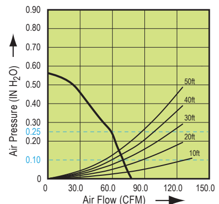
70BT Fan Curve
